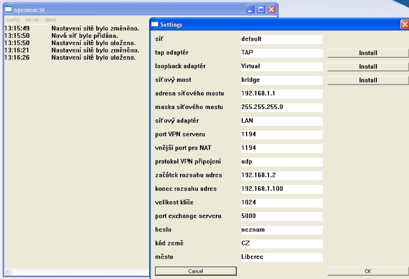
Obr. 1. ukázka GUI aplikace
