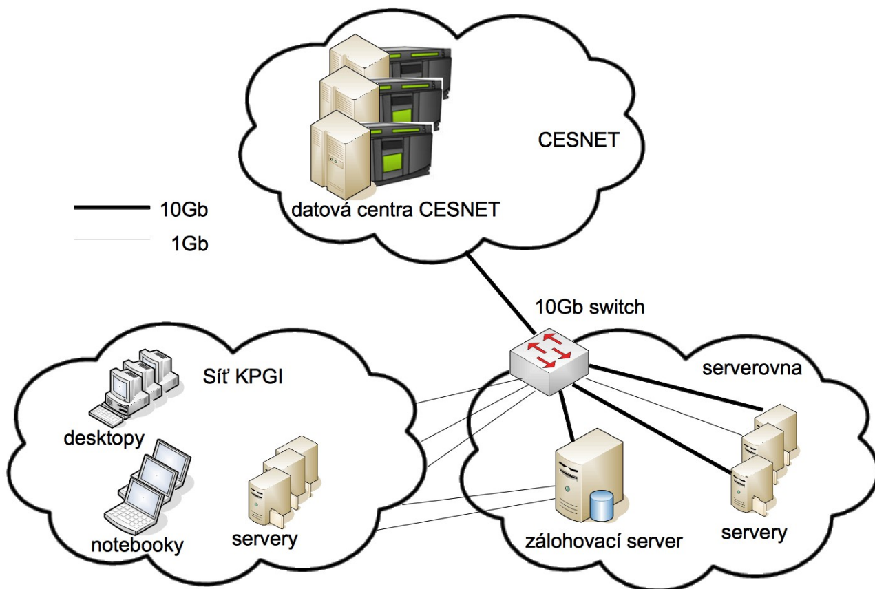
Obrázek 1: Zapojení pracoviště
